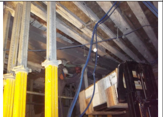
Foto 3 – Reforço com Vigamento Metálico
